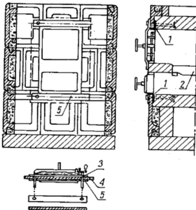
Rys. nr 5: 1- pas izolacji, 2-ruszt, 3- rura drzwiczekowa, 4-płyta czołowa, 5-podkładka oporowa
