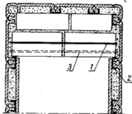
Rys. nr 4: 1- opaski z drutu \varnothing 3 mm, 2- klamerki, 3- pręt \varnothing 7 mm
